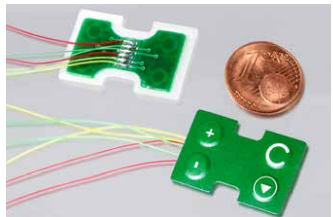
Miniatur-Folientastatur als Baugruppe mit Leiterplatte und Kabelanschluss
