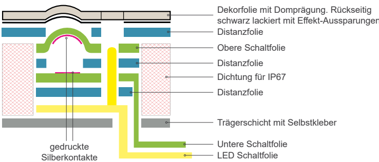
AUFBAU MIT 8 FOLIEN & TASTENPRÄGUNG
