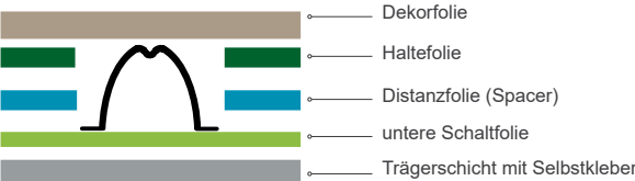
AUFBAU MIT METALLSCHNAPPSCHEIBEN
